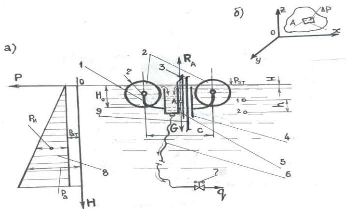
Рисунок 2. Схема к расчету поплавкового дозатора:
