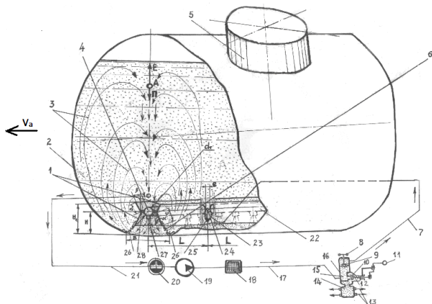
Рисунок 1 - Схема технологического процесса работы предлагаемой виброгидромешалки:
